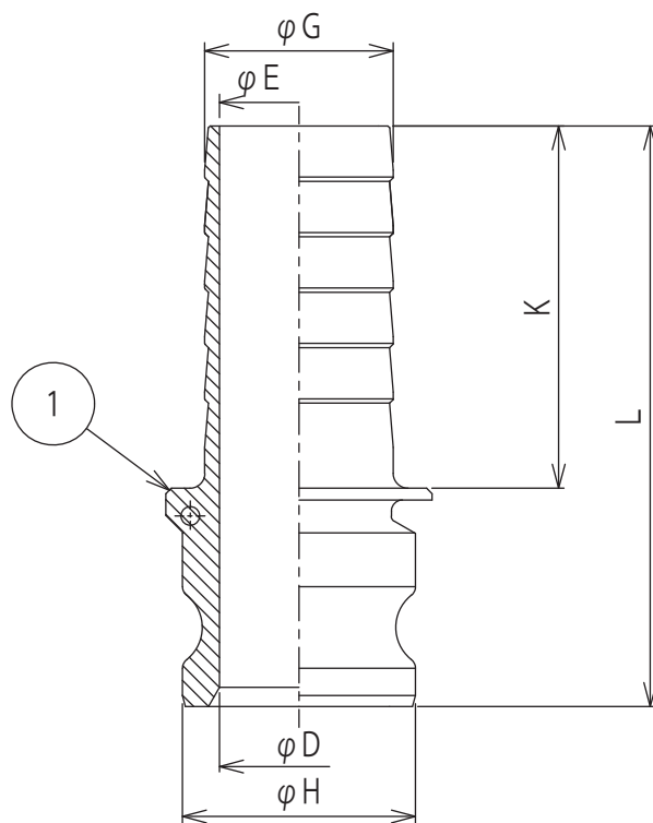
633-ET AL サイズ別寸法表 (単位: mm)
