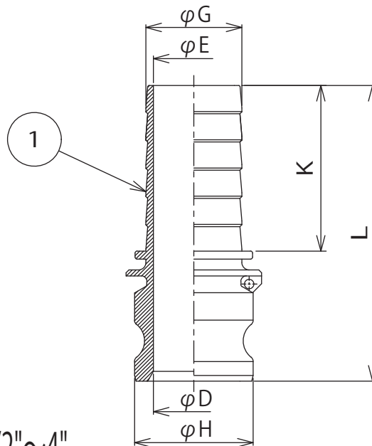
633-ET SST サイズ別寸法表(単位：mm)
