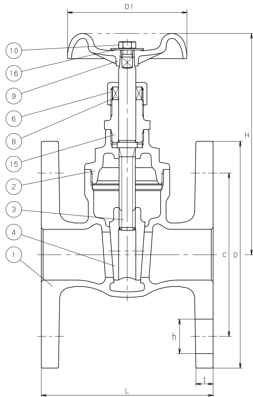
寸法表
