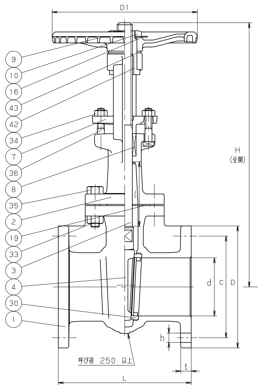
寸法表
