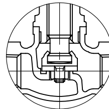
呼び径 1/4 のみ
