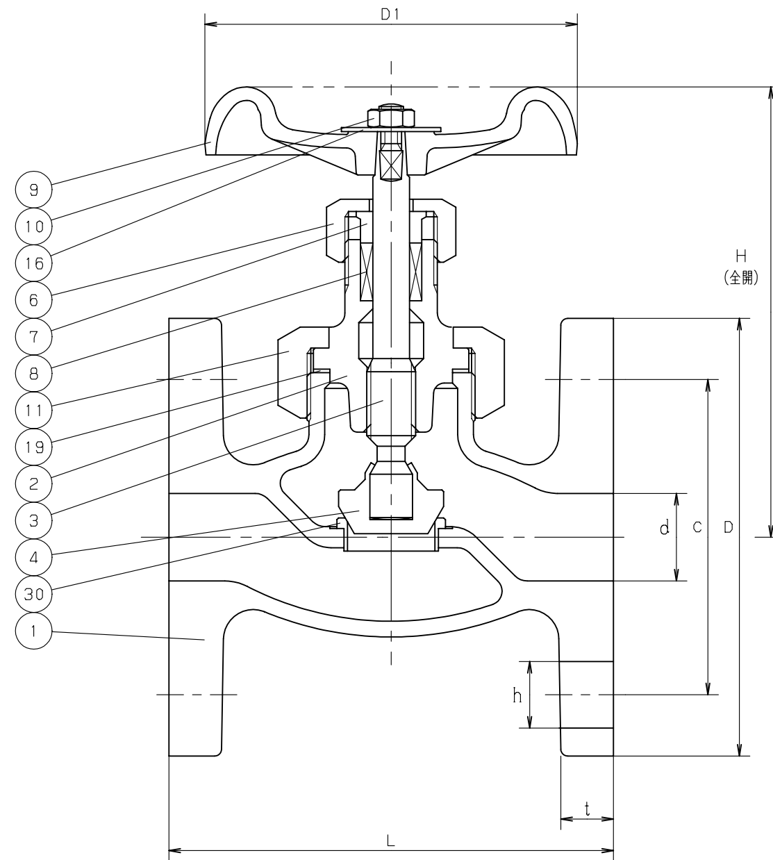
寸法表
