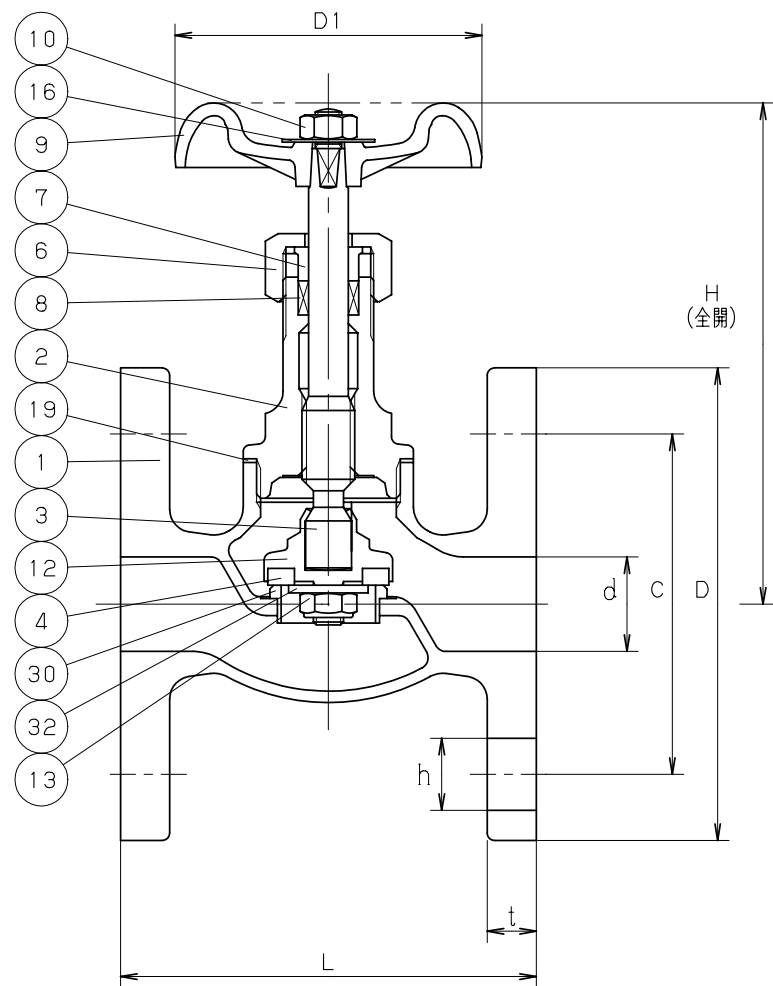
寸法表
