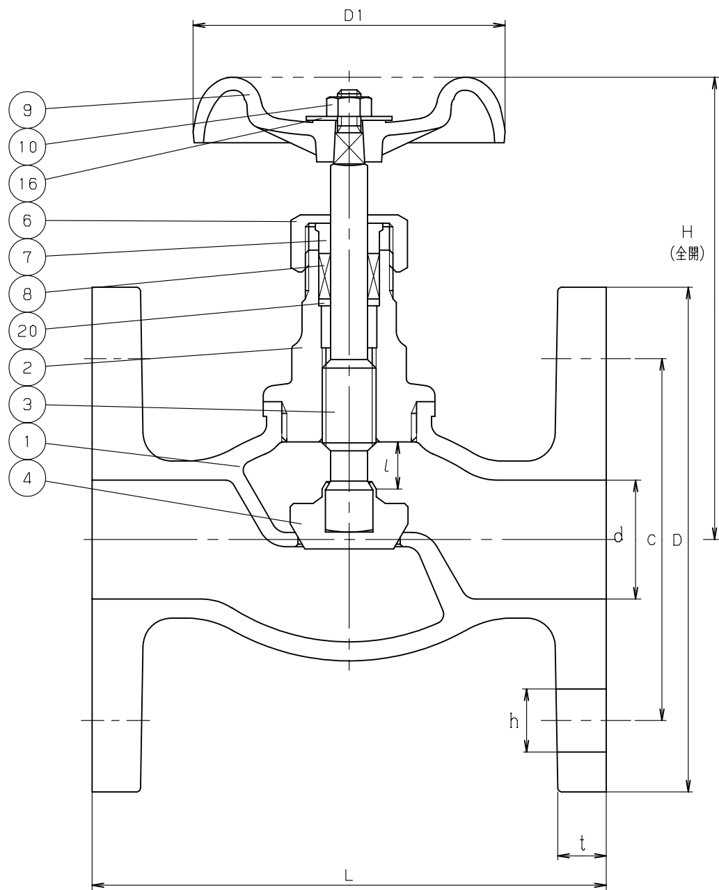
寸法表
