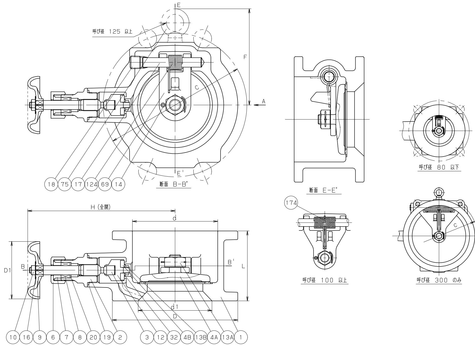
寸法表
